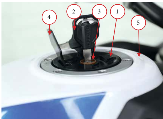
Фото 2.21. Крышка топливного бака модели ZT125-Z2 и ZT350-S:
