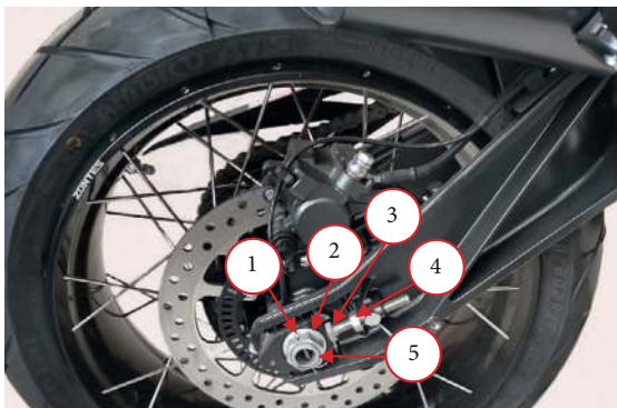
Фото 4.14. Снятие заднего колеса (вариант): 1 – шплинт; 2 – гайка оси колеса; 3 – натяжитель цепи; 4 – стопорная гайка; 5 – ось колеса.
