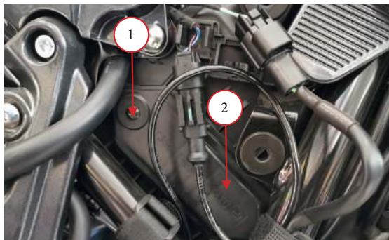
Фото 4.1. Снятие воздушного фильтра: 1 – винт крепления крышки; 2 – крышка фильтра; 3 – воздушный фильтр; 4 – скобка корпуса фильтра.
