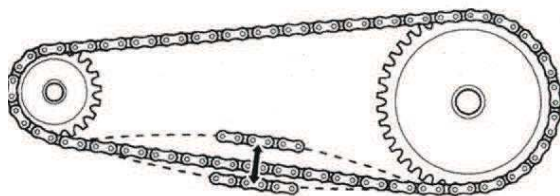
Рисунок 3. Натяжение цепи.
