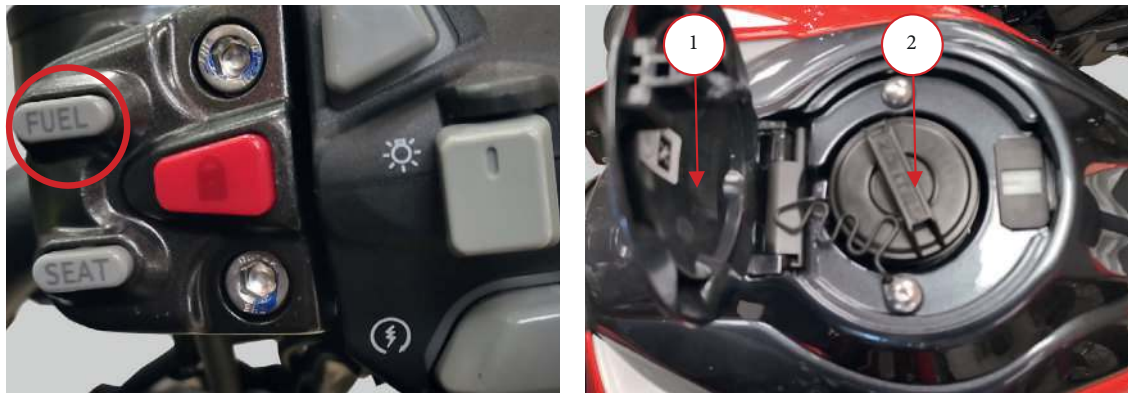
Фото 2.22. Открывание крышки топливного бака моделей ZT125-U/U1, ZT350-R/R1, ZT350-X/X1, ZT350-T, ZT350-GK, ZT350-VX, ZT350-V1 (с бесключевым доступом): «FUEL» - кнопка открытия внешней откидной крышки; 1 - внешняя защитная крышка; 2 - крышка топливного бака.
